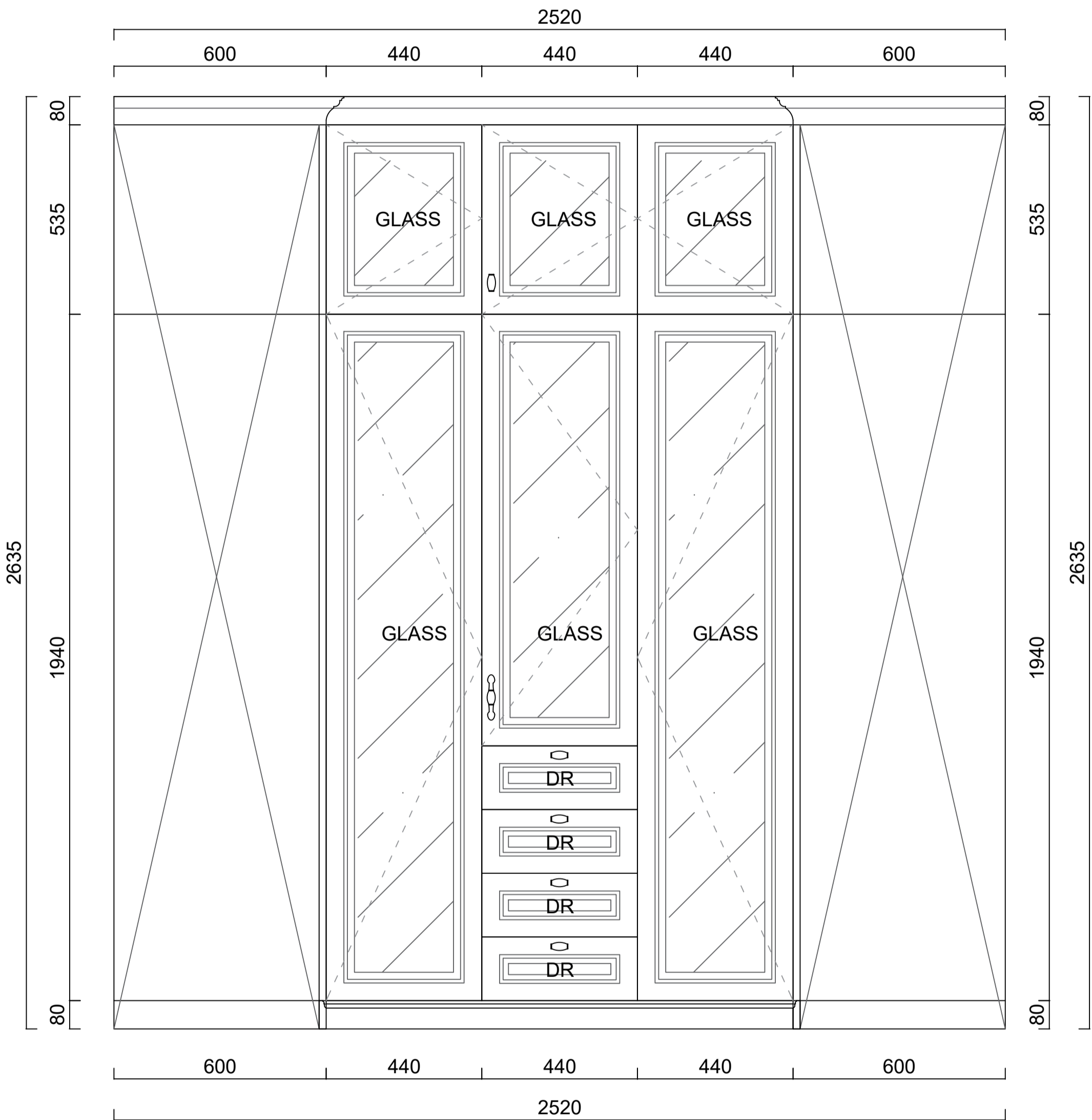
B ELEVATION
