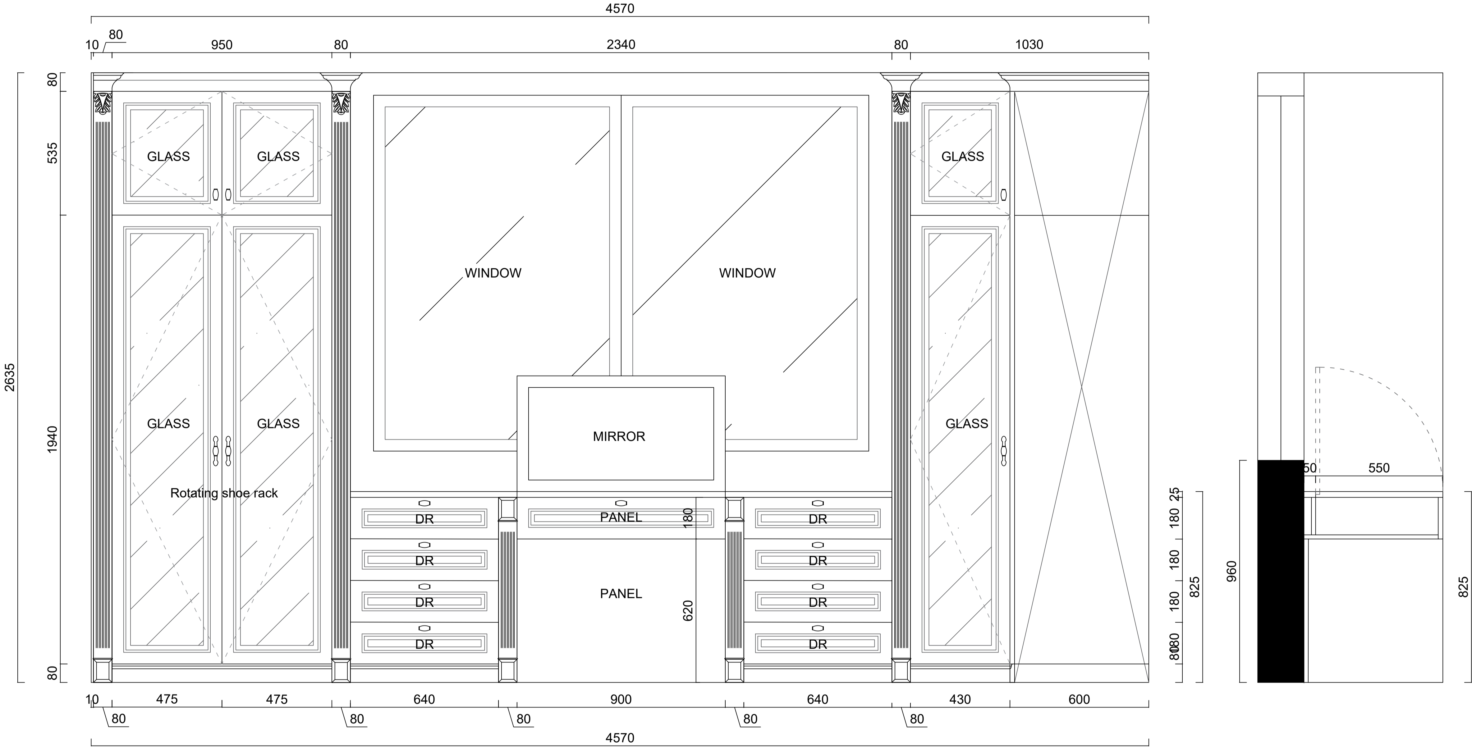
A ELEVATION
