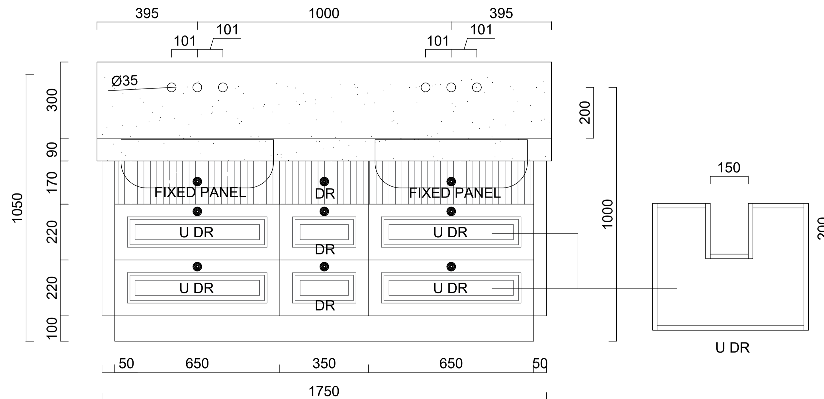
ELEVATION
