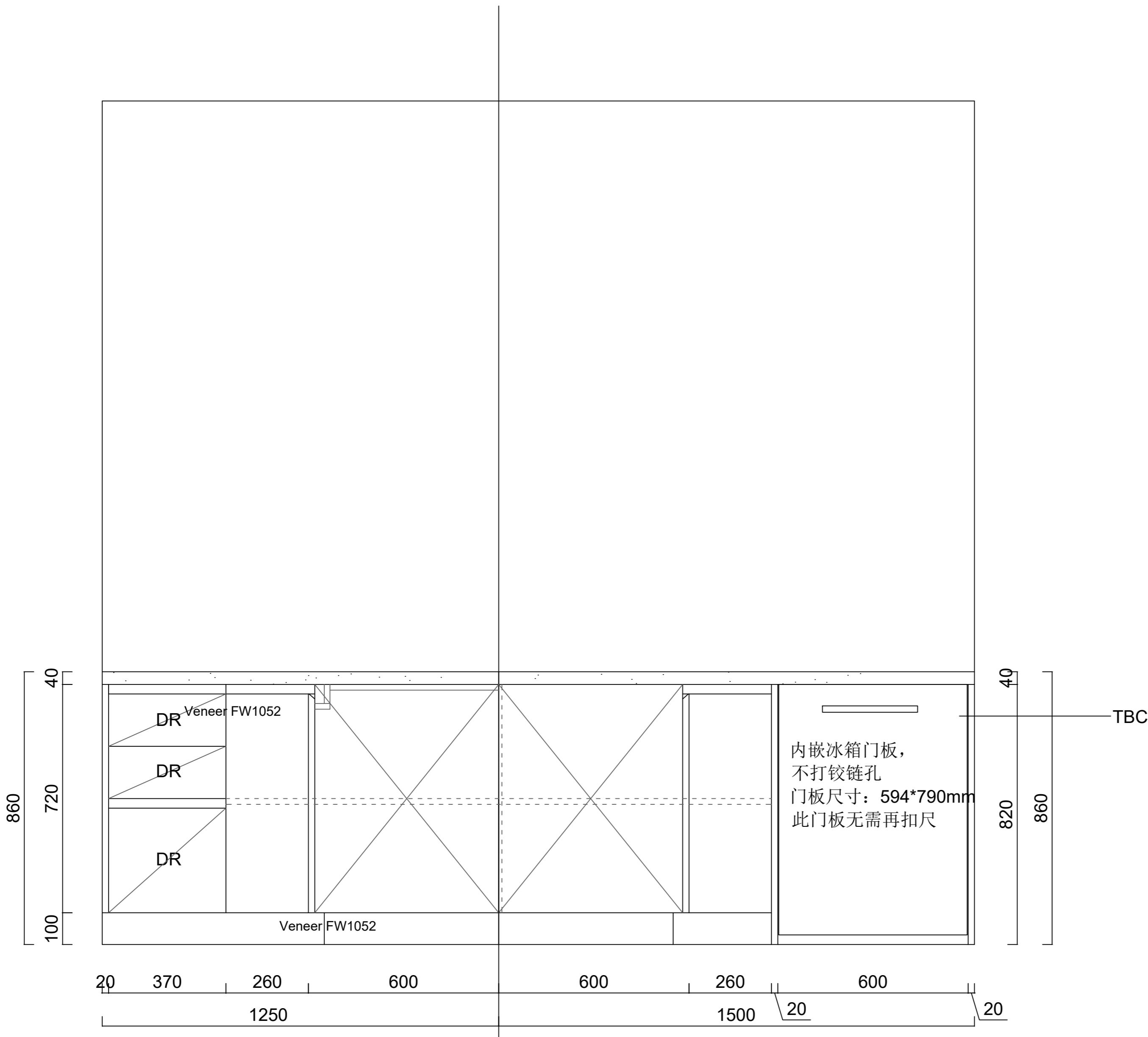
A ELEVATION
