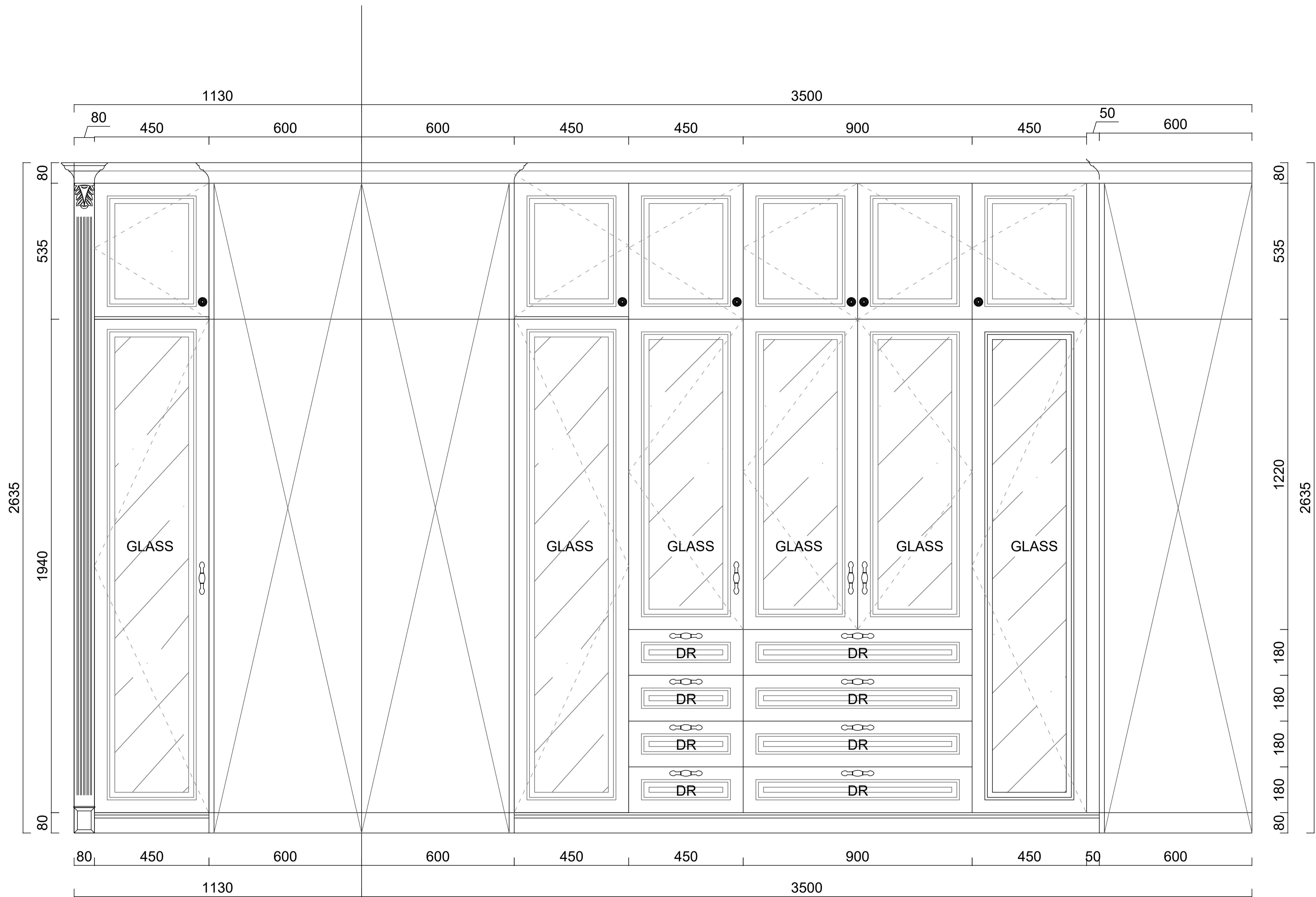
A ELEVATION
