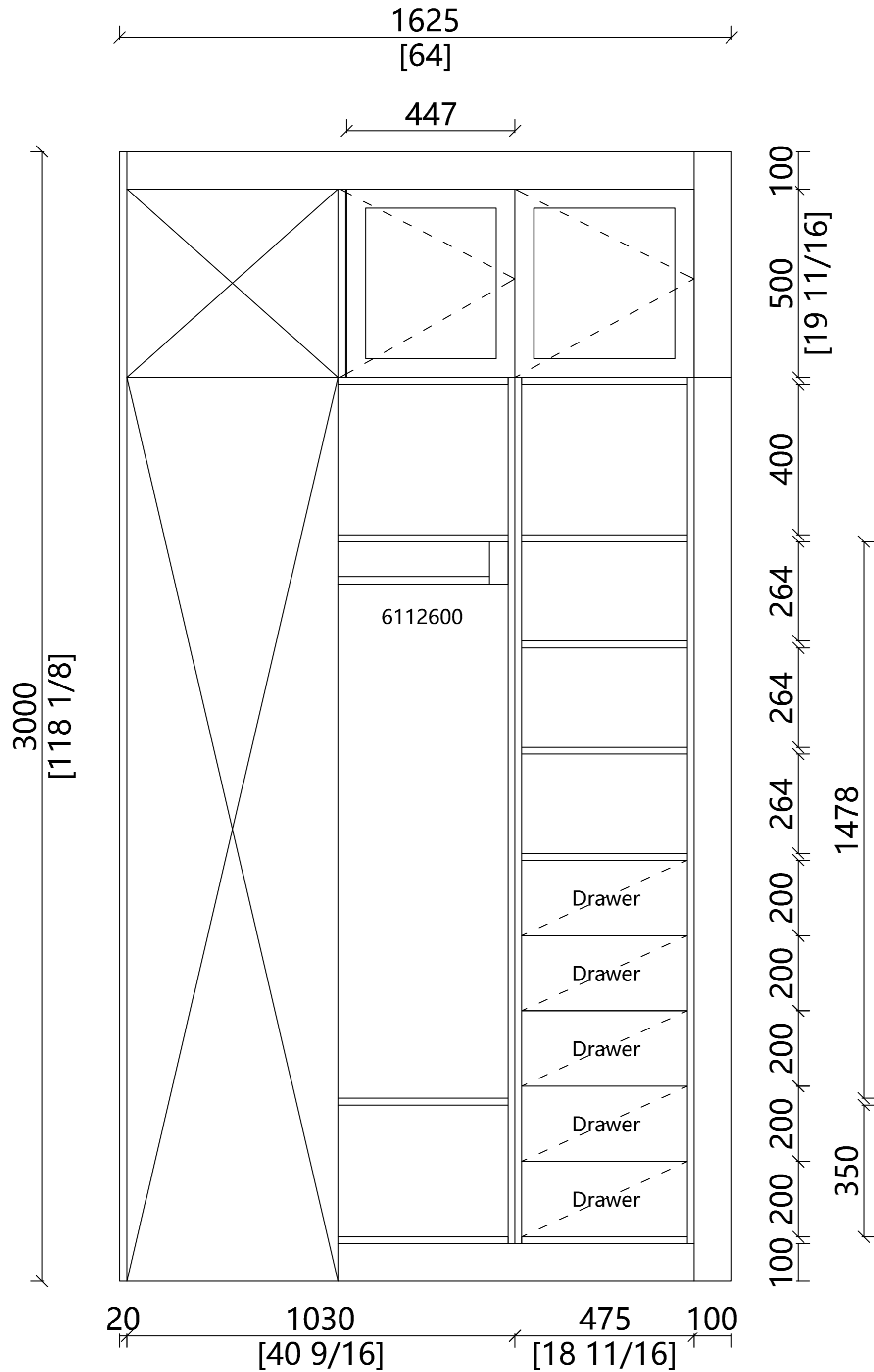
ELEVATION B
