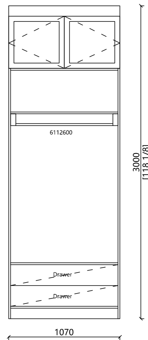
ELEVATION B
