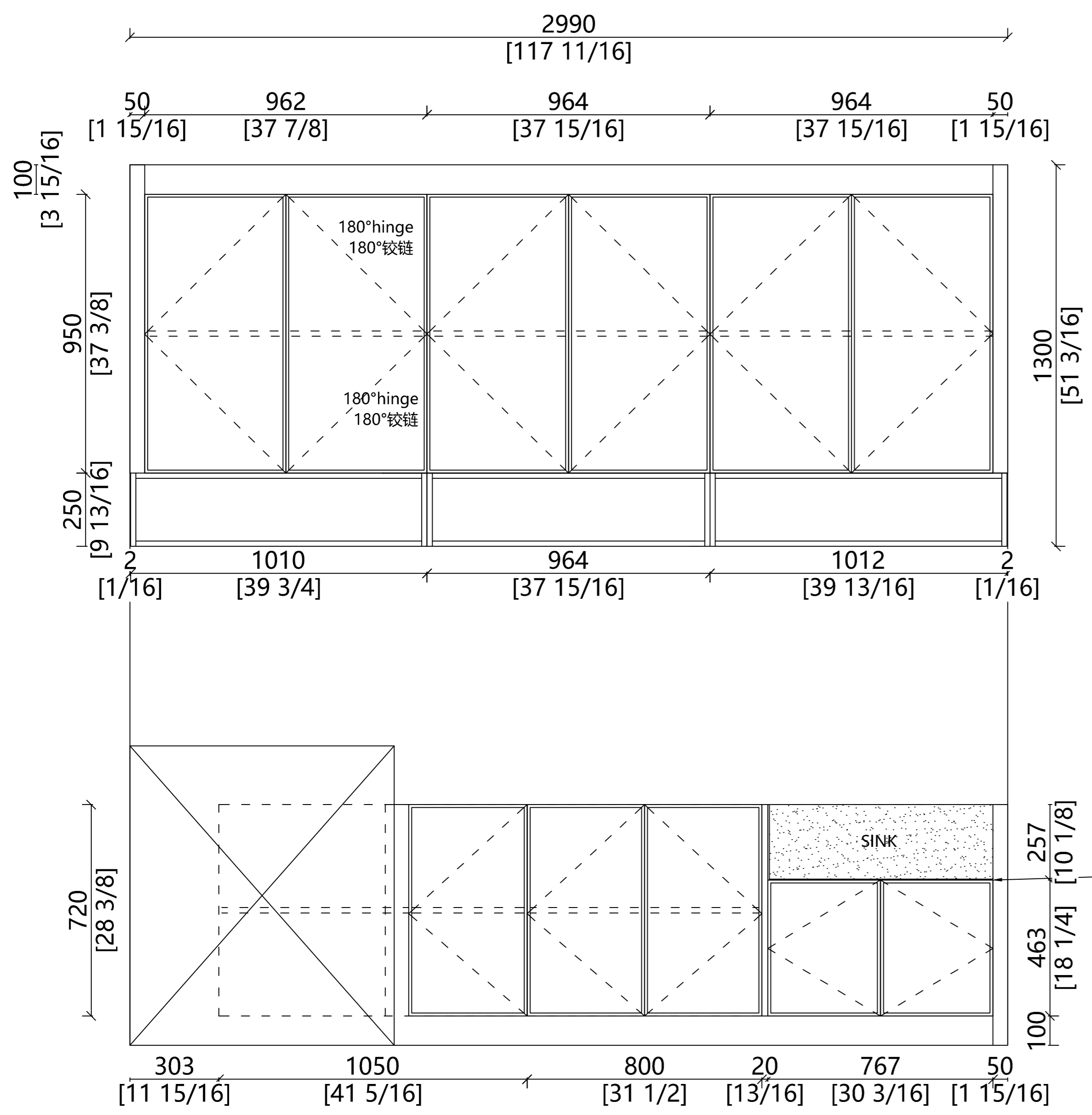
ELEVATION A
