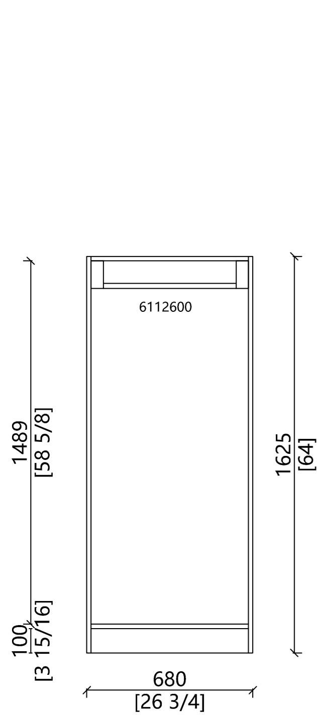
ELEVATION A
