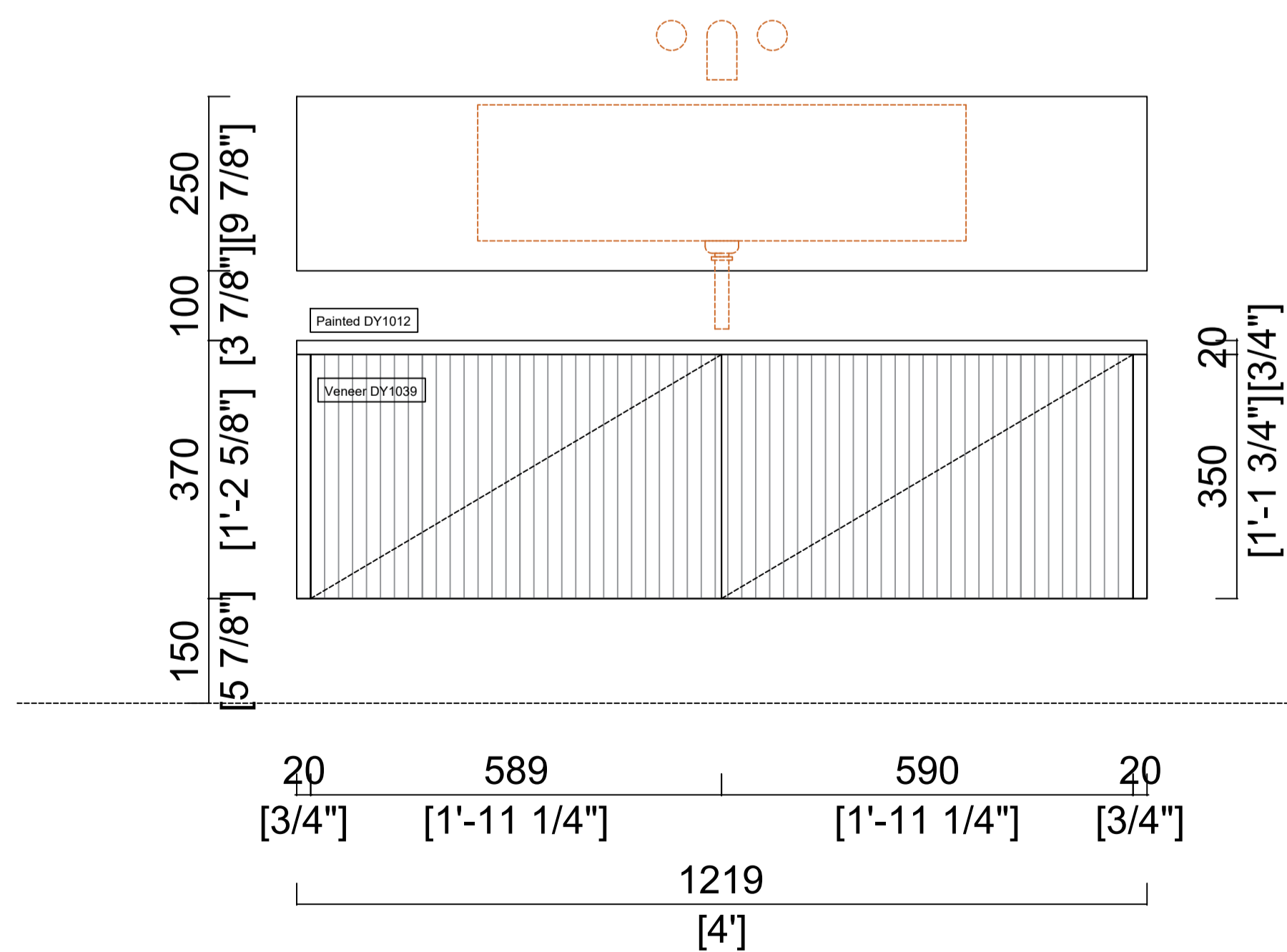
ELEVATION
