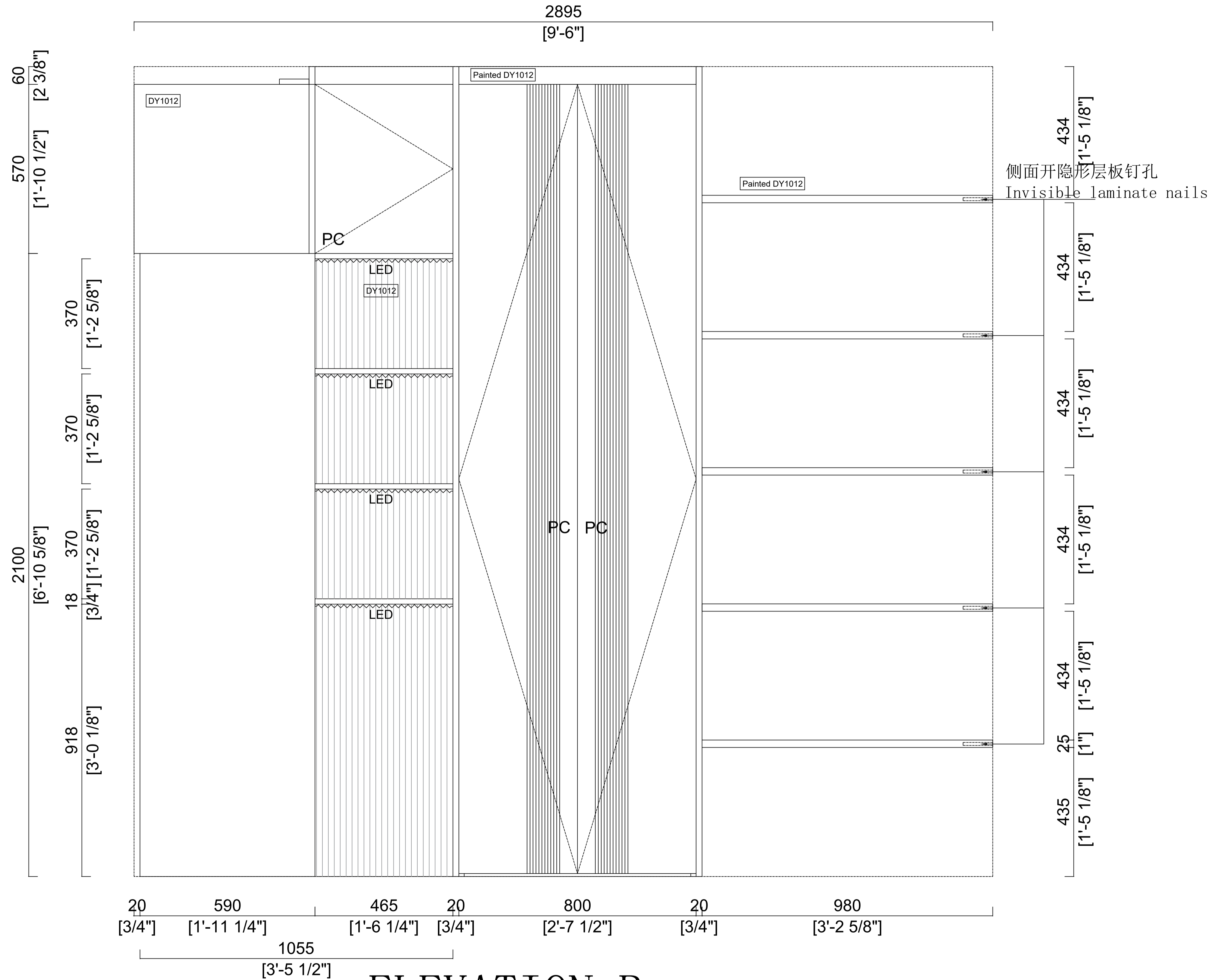
ELEVATION B
