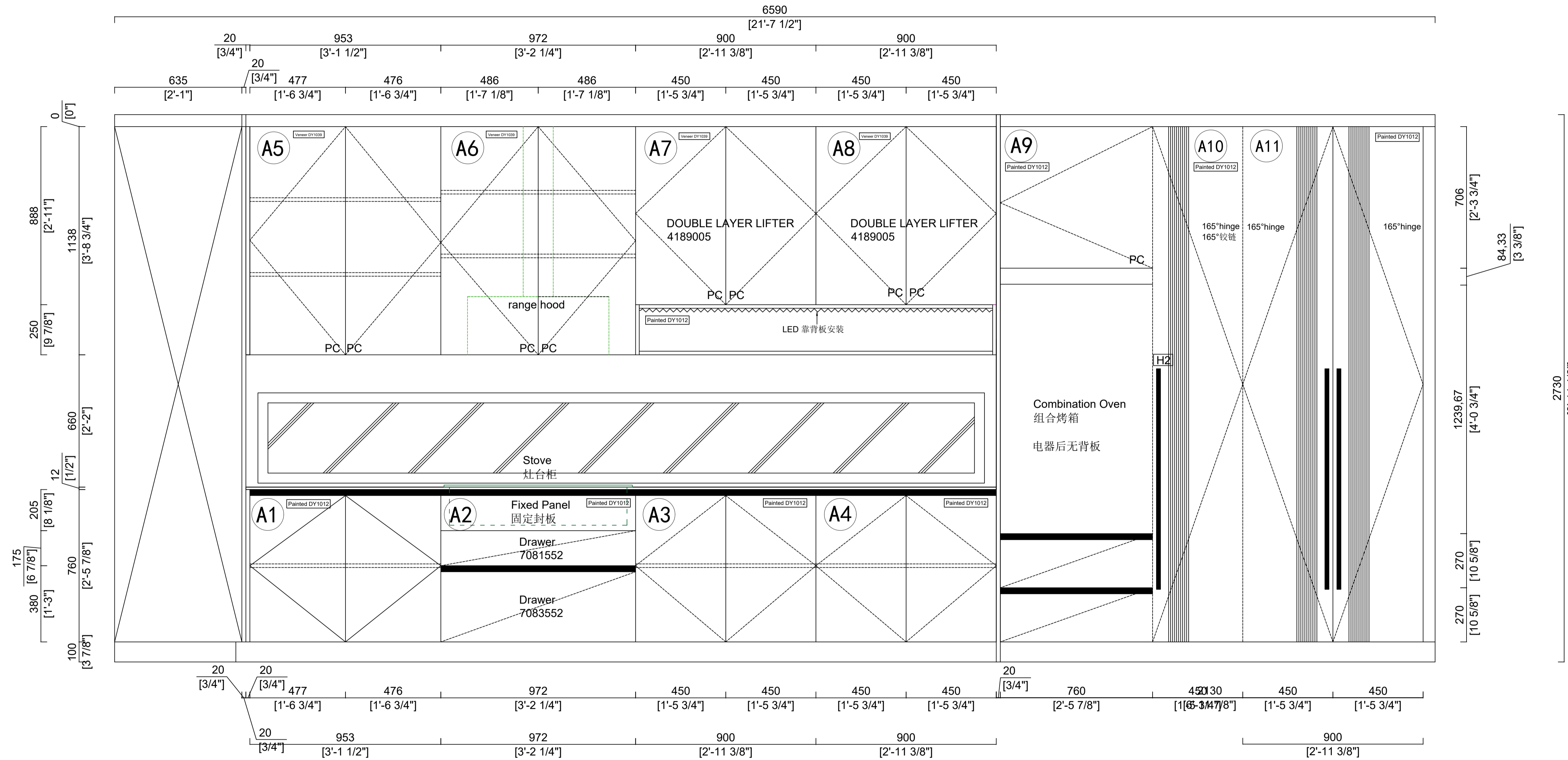
ELEVATION A
