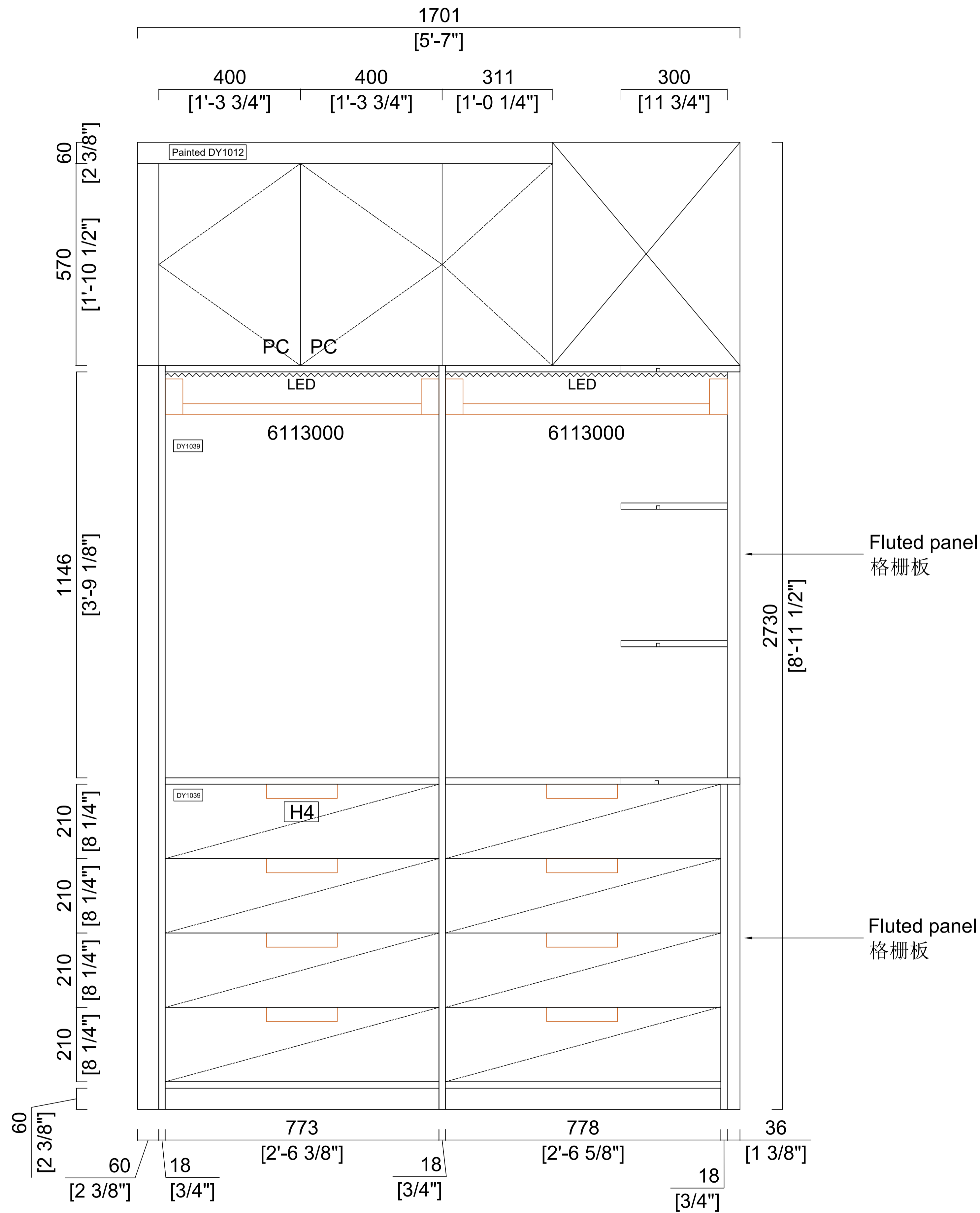
ELEVATION A
