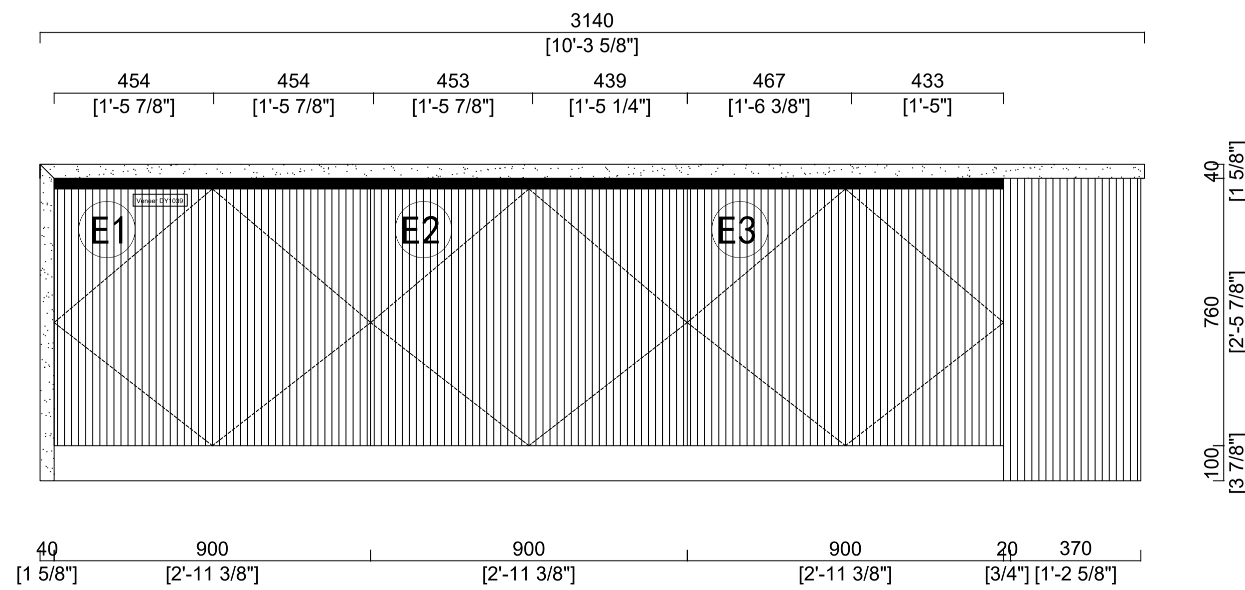
ELEVATION E
